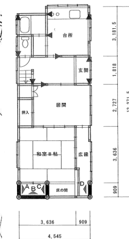
1 階平面図 1/100
