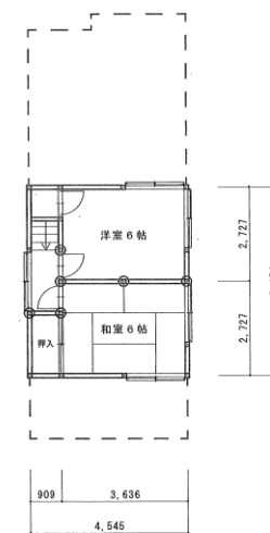
2 階平面図 1/100
